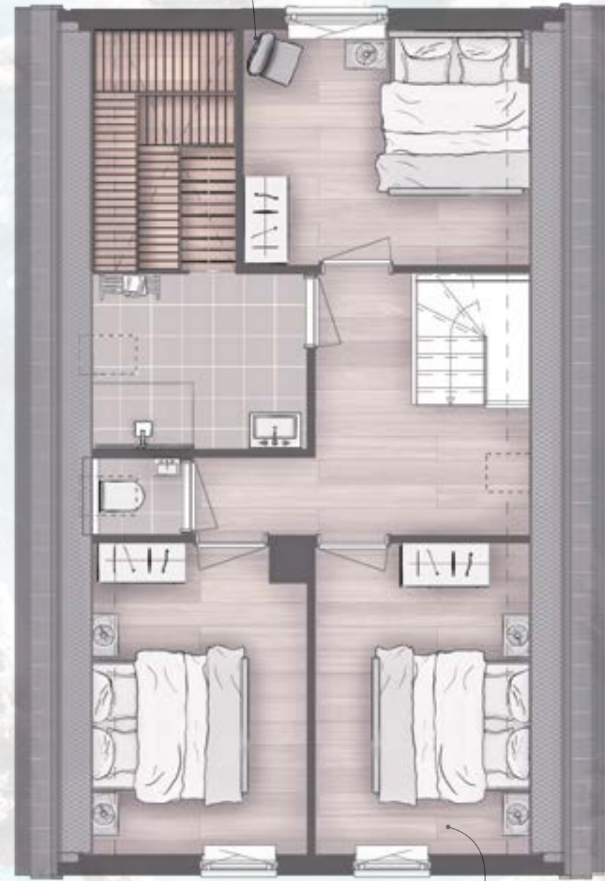
Eerste verdieping
